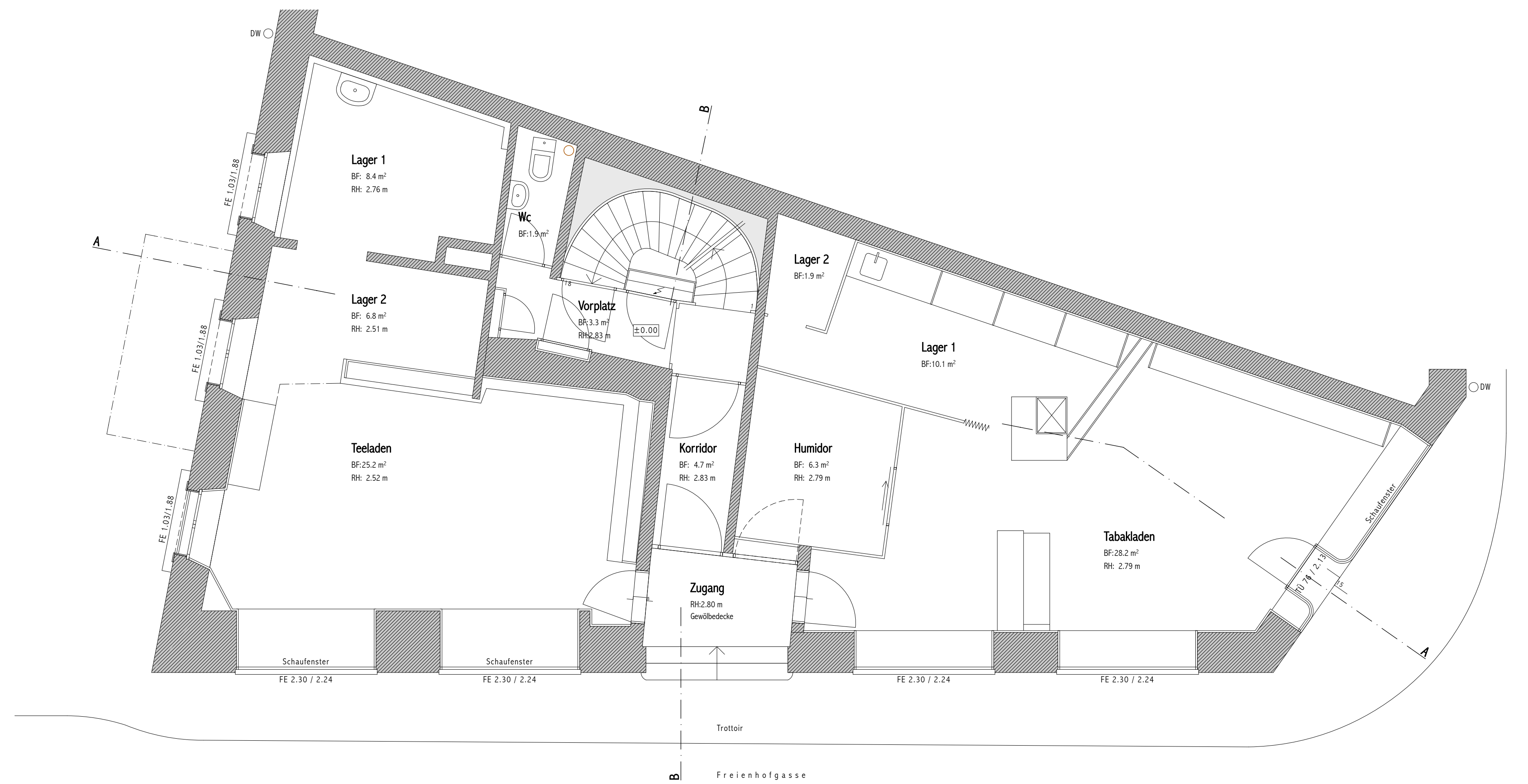
Erdgeschoss
